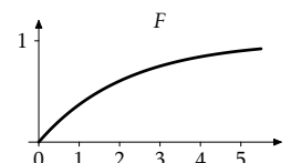
Tæthedsfunktion og fordelingsfunktion for eksponentialfordelingen med \beta = 2.163 .
